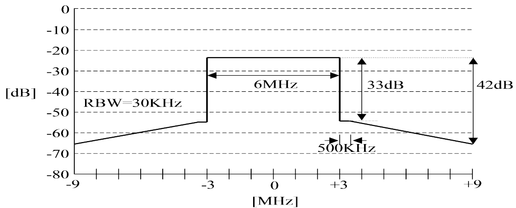
인접채널 감쇠특성
